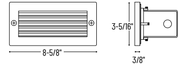
NSW-841/32 Louver
