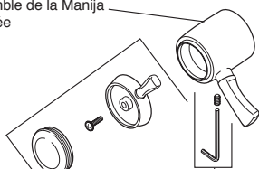
RP50465 Set Screw & Wrench Tornillo de Ajuste y Llave Vis de calage et Clé
